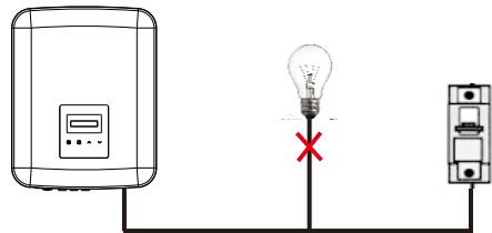
Connessione errata tra carichi e inverter
